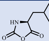
Leu-NCA
