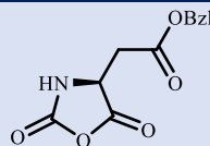
Asp(OBzl)-NCA
